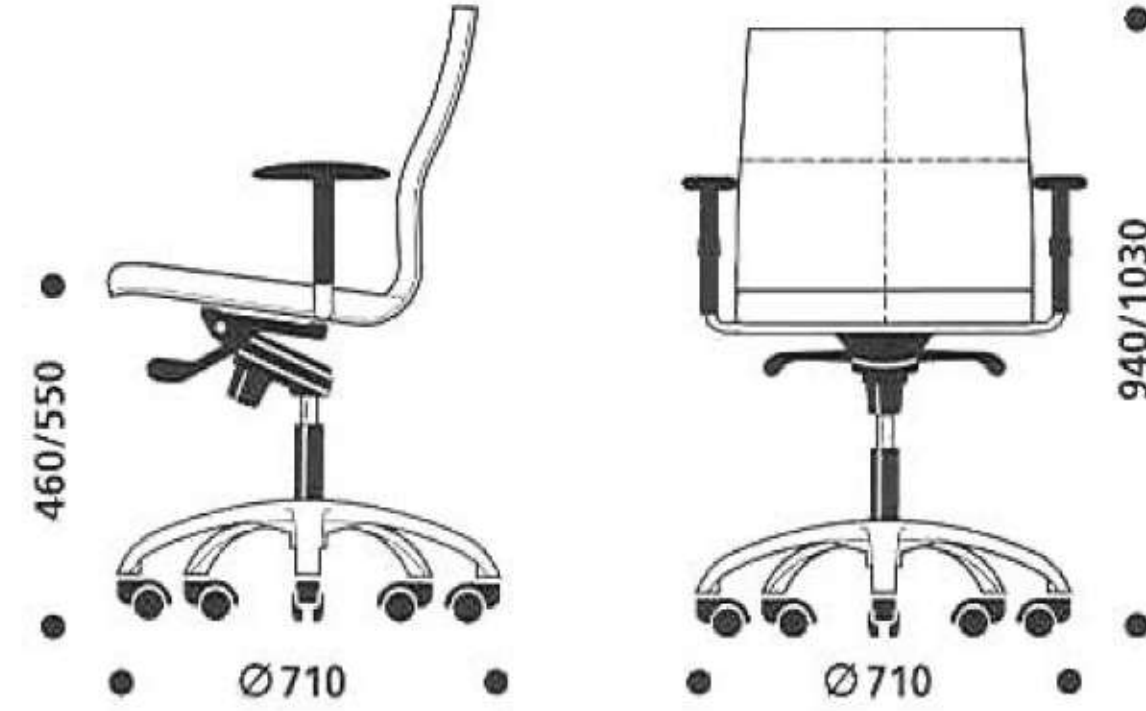
BOSS 10.026 B Sillón respaldo bajo. Giratorio. Gas. Brazos regulables.
