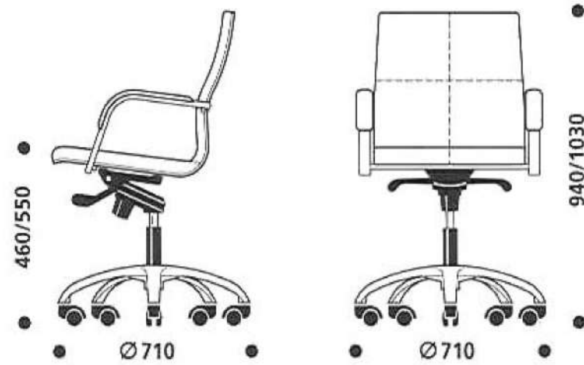
BOSS 10.025 B Sillón respaldo bajo. Giratorio. Gas. Brazos fijos.
